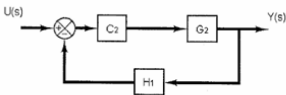
Figura do 2: Diagrama de blocos que relaciona Y(s) com U(s) .
